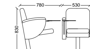
Schienale arrotondato fianco sospeso con tavoletta Round backrest on the suspended bench side with writing board
